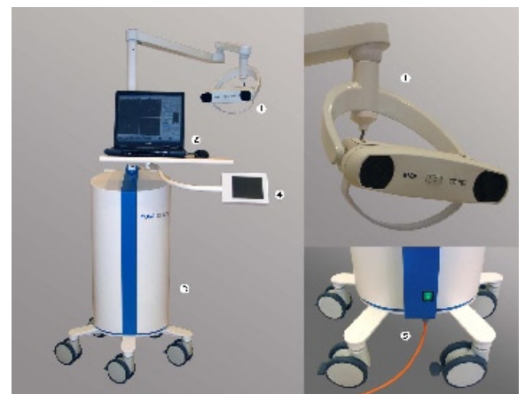
Abb. 1: Das neue Planungs- und Navigationssystem MONA_DENT® mit seinen Komponenten: Infrarot-Kamera (1), Notebook (2), Chassis (3), 5" TFT-Display (4), standfestes Drehgestell (5).
